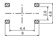
P. C. B. Layout
