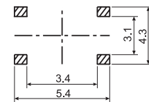
P. C. B. Layout
